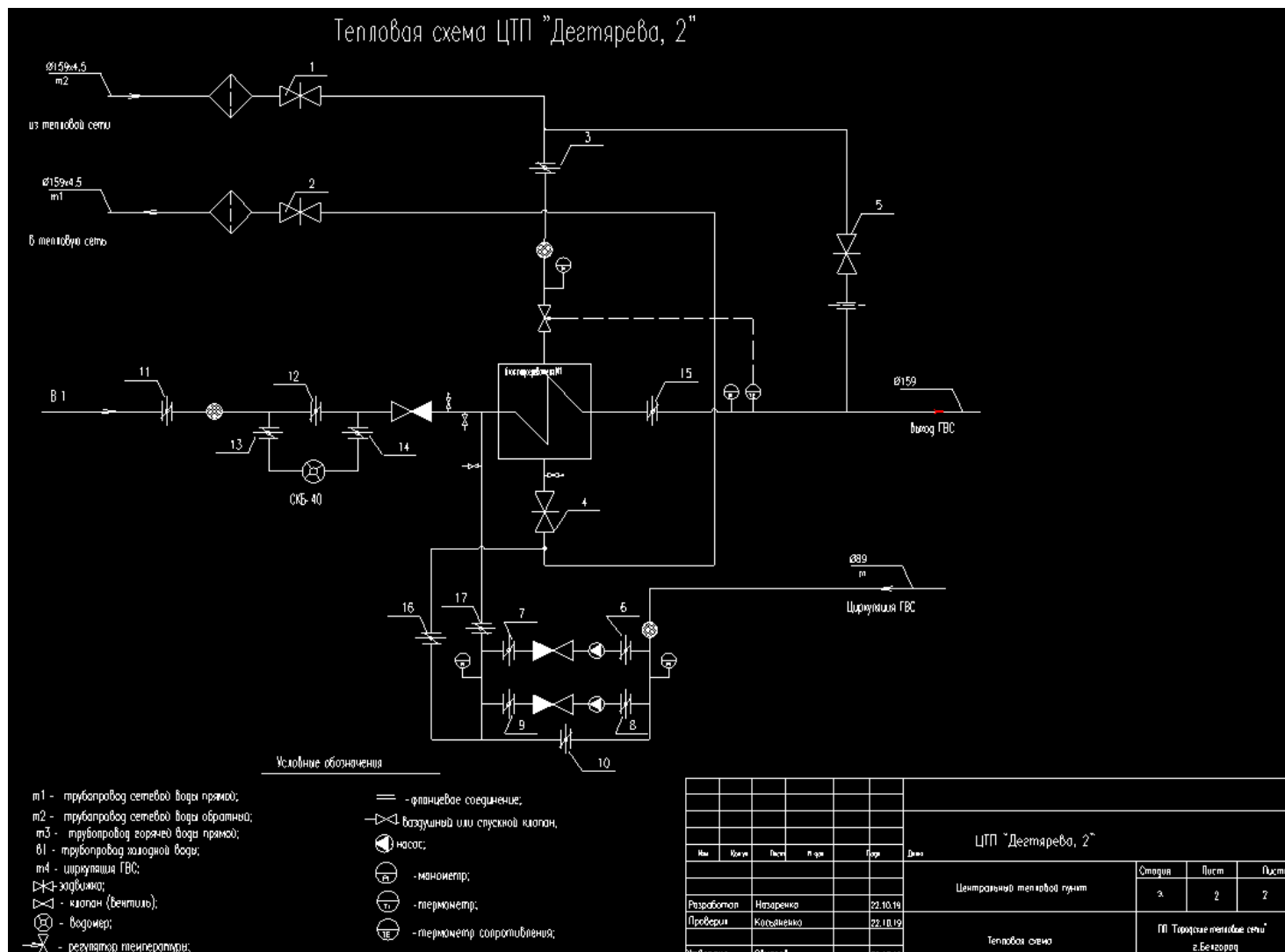
Рисунок 1.8.40 Принципиальная схема теплового пункта «Дегтярева, д. 2»
