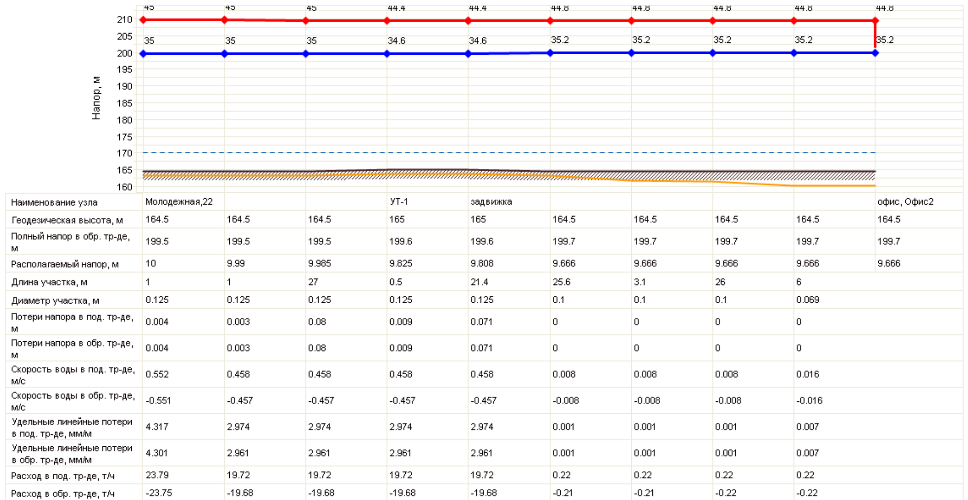
Рисунок 1.9.49 Пьезометрический график котельной «Молодежная, д. 22»
