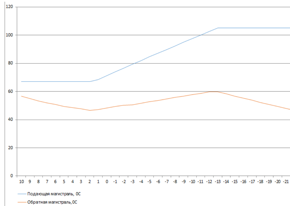
Рисунок 5.1 Температурный график «Белгородская ТЭЦ»
