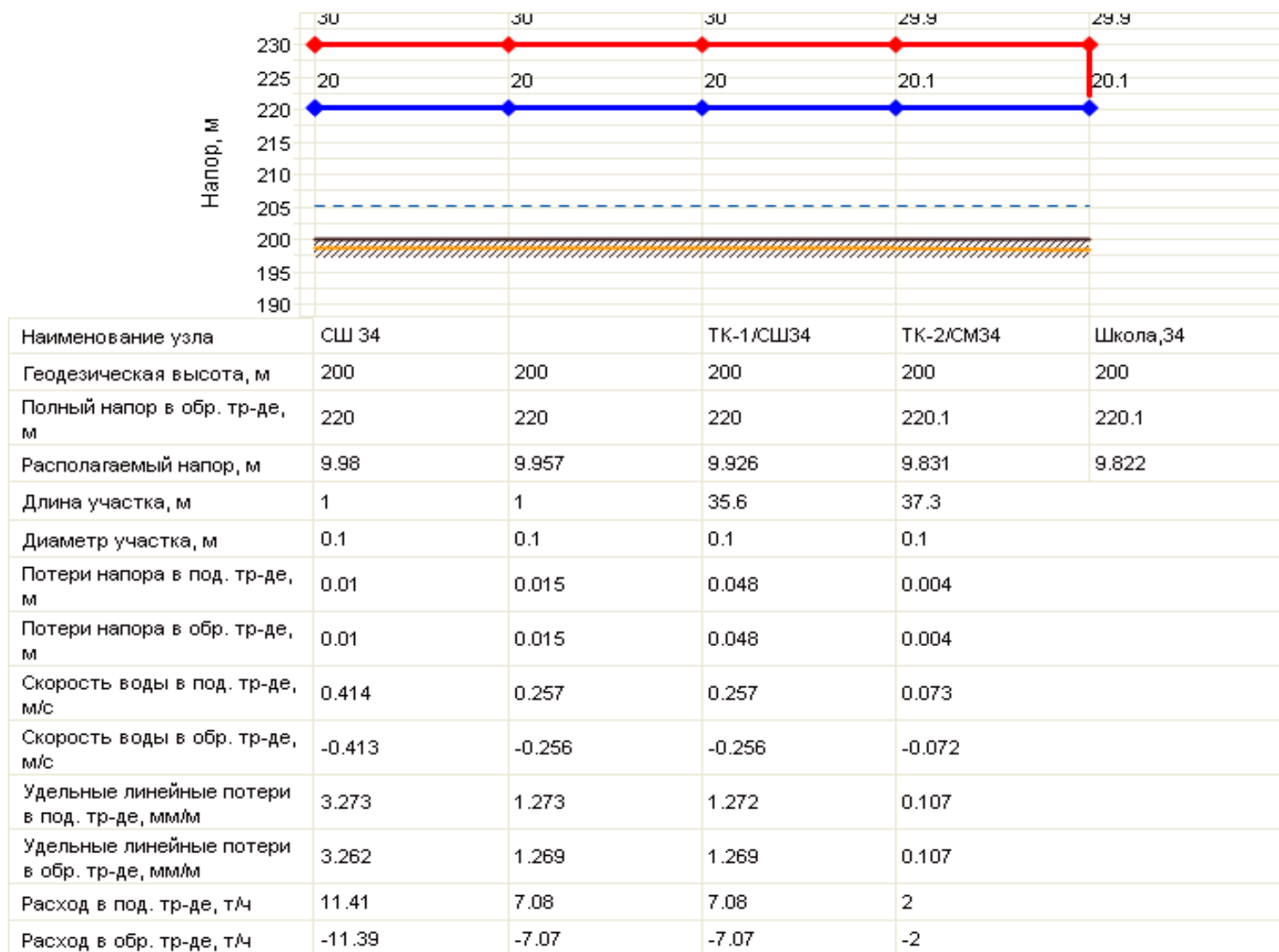
Рис. 1.9.64 Пьезометрический график котельной «Школа, № 34»
