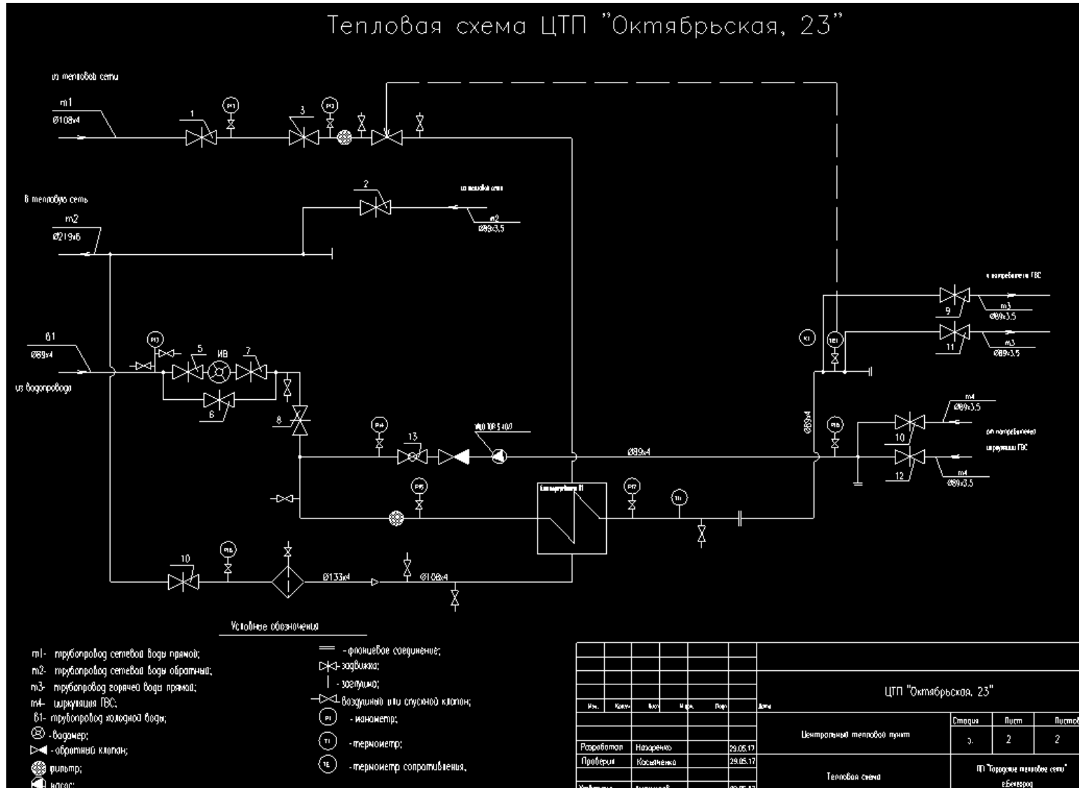
Рисунок 1.8.49 Принципиальная схема теплового пункта «Октябрьская, д. 23»
