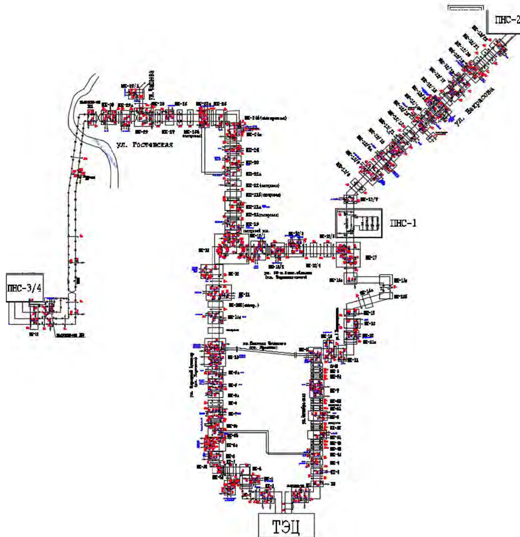
Рисунок 1.9.1 Схема магистральных сетей от ТЭЦ г.Белгорода
