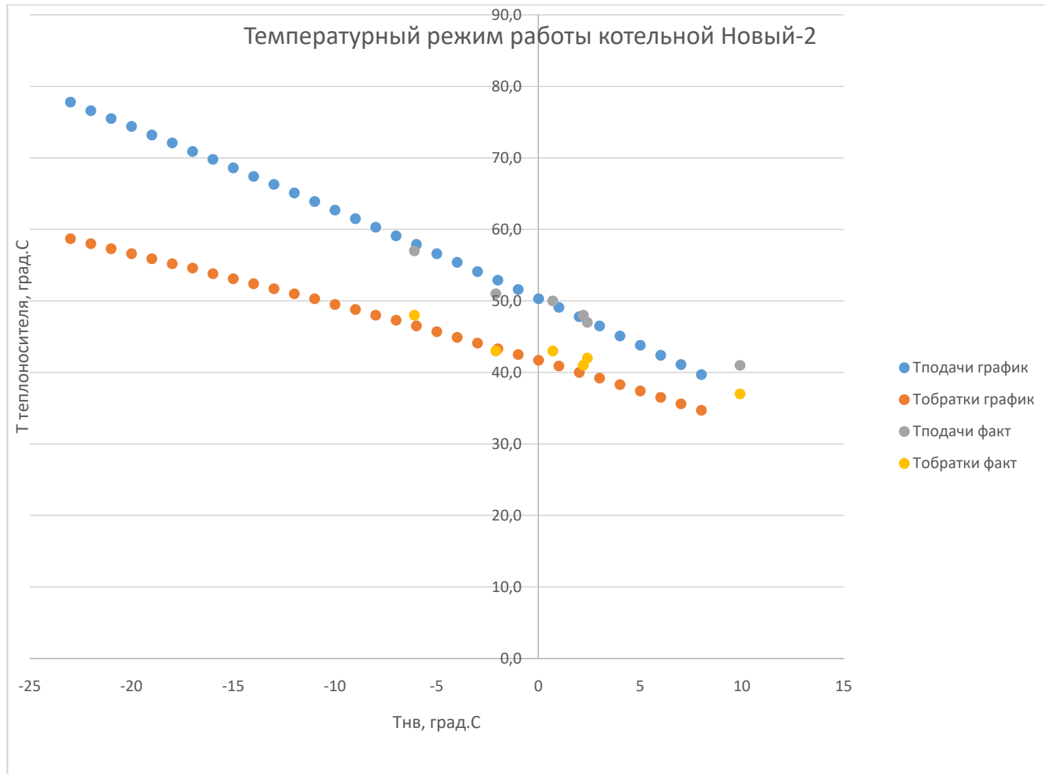
Рисунок 1.9.77 Температурные режимы котельных: Почтовая, Новый-2
