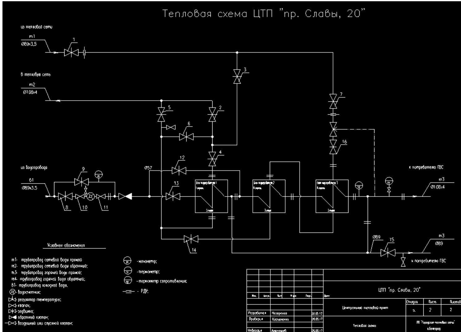
Рисунок 1.8.23 Принципиальная схема теплового пункта «Славы, 20»
