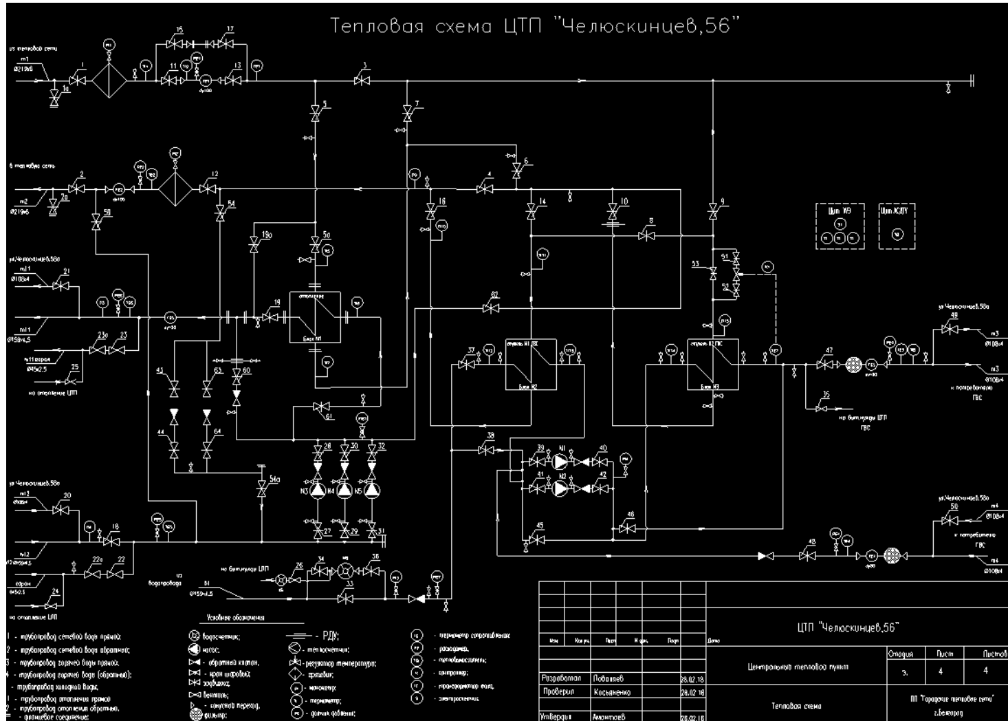
Рисунок 1.8.18 Принципиальная схема теплового пункта «Челюскинцев, 56»
