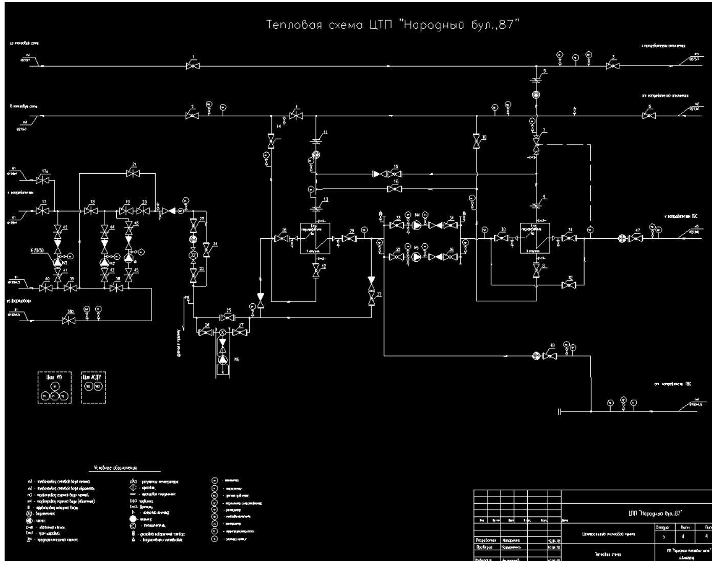
Рисунок 1.8.46 Принципиальная схема теплового пункта «Н. Бульвар, д. 87»
