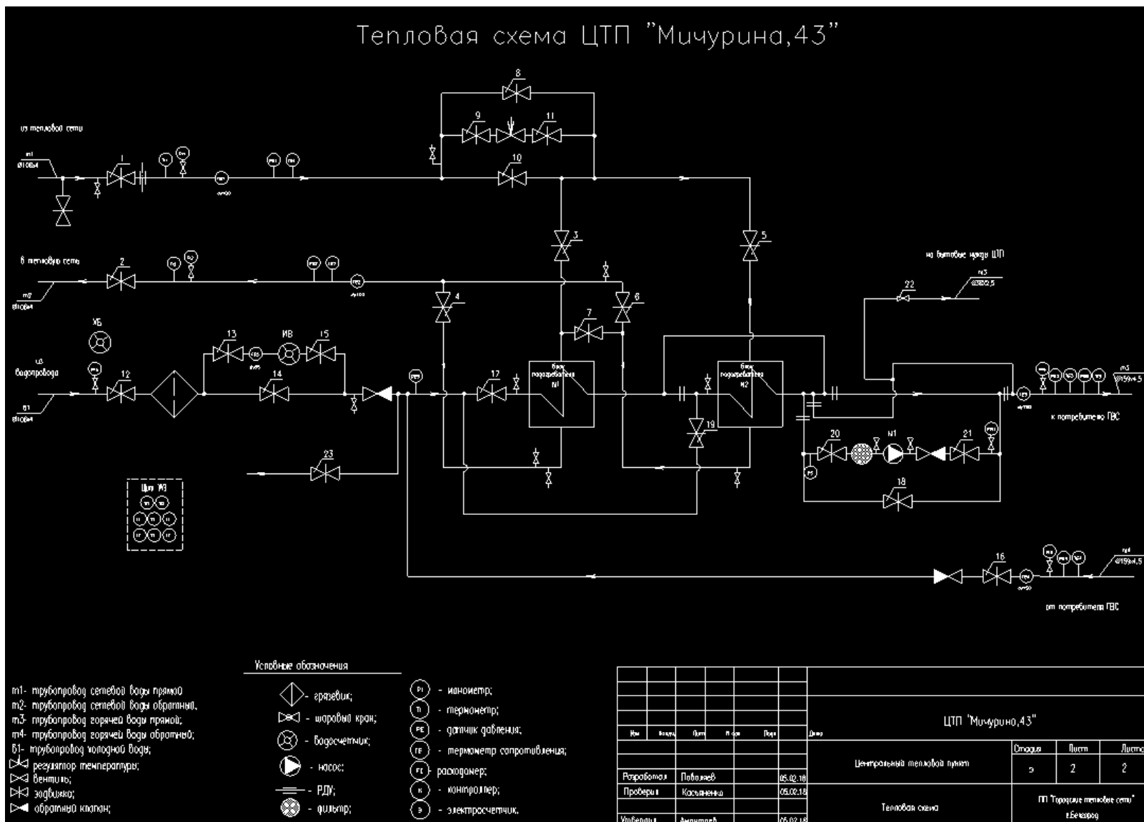
Рисунок 1.8.10 Принципиальная схема теплового пункта «Мичурина, д. 43»
