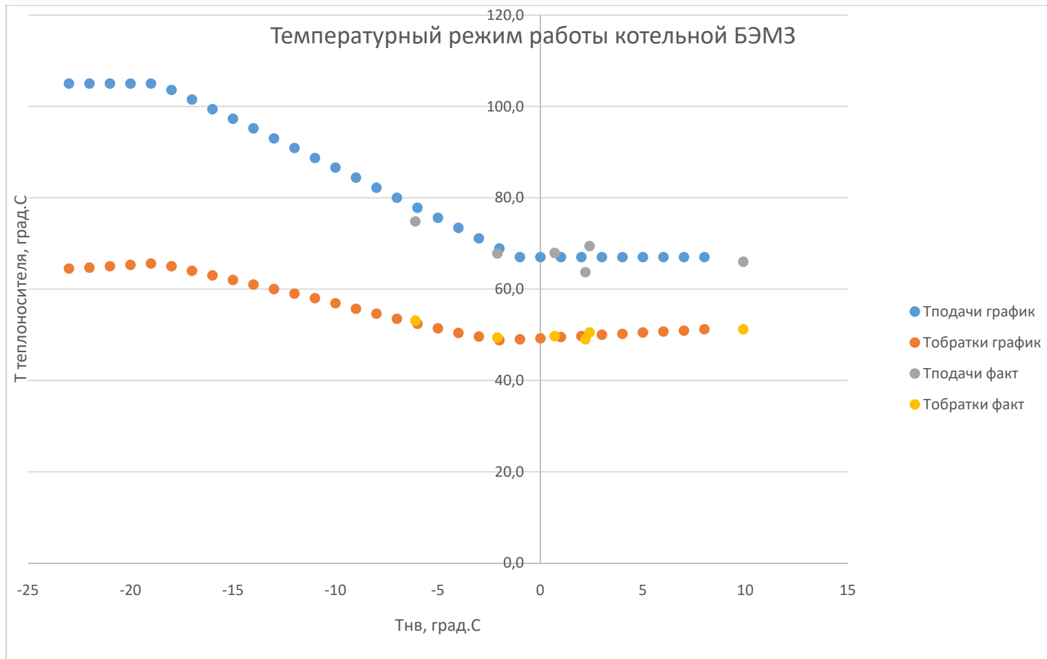
Рисунок 1.9.74 Температурные режимы котельных: 1 СМР, 2 СМР, БЭМЗ, Сокол
