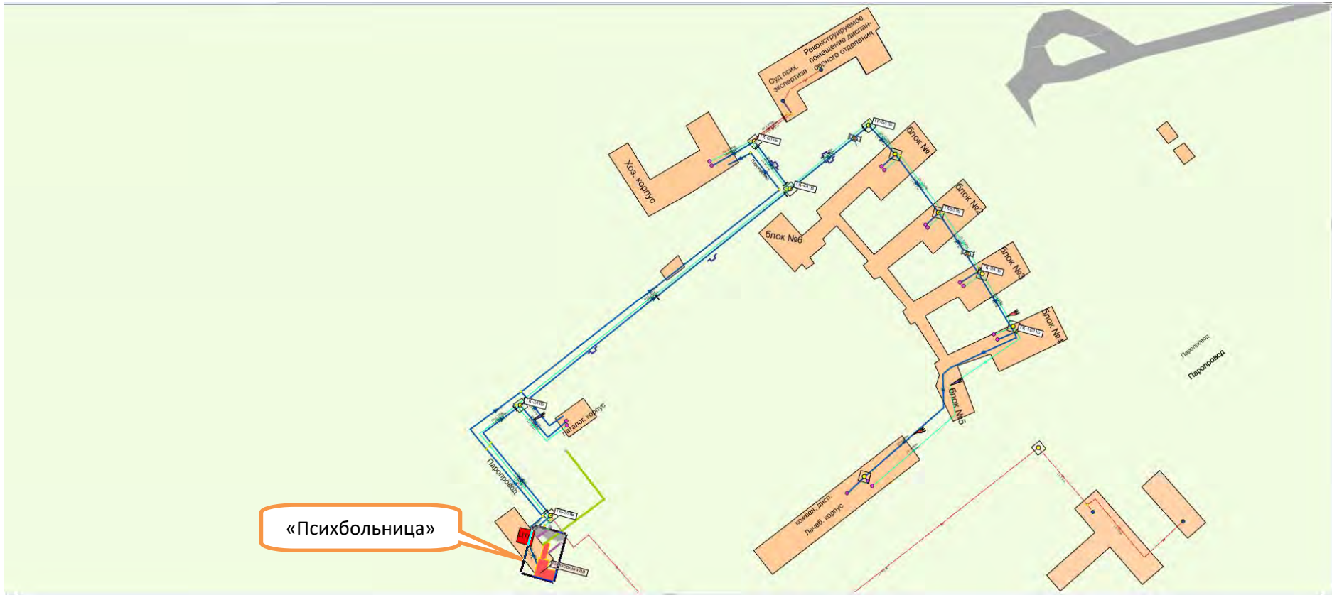
Рисунок 1.9.13 Схема магистральных сетей от котельной «Psikhbol'nitsa»
