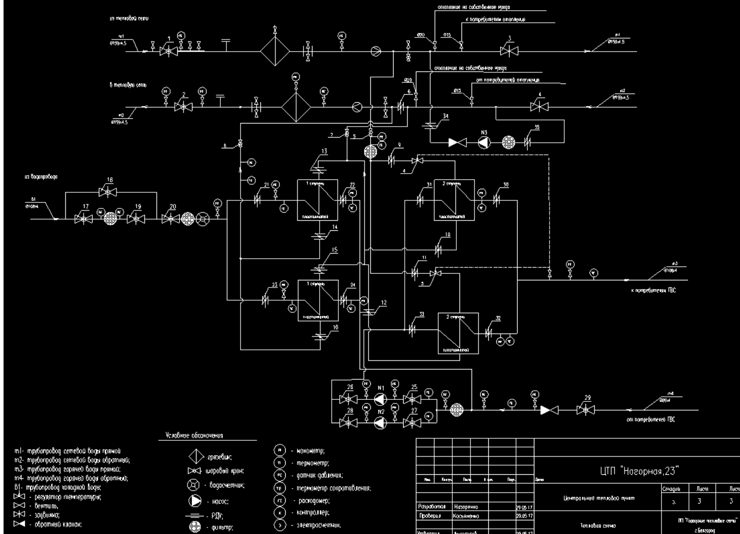
Рисунок 1.8.45 Принципиальная схема теплового пункта «Нагорная, д. 23»
