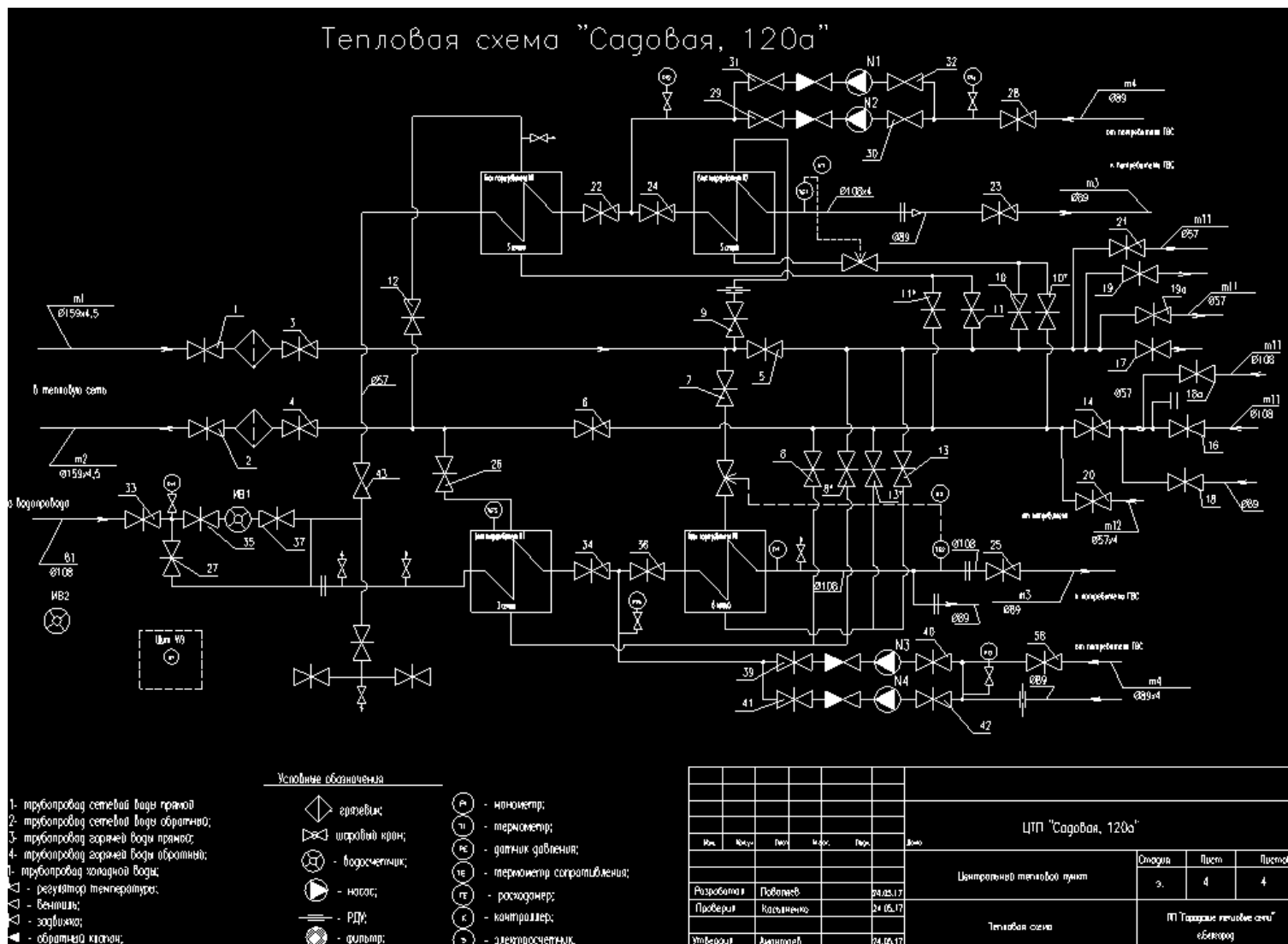
Рисунок 1.8.13 Принципиальная схема теплового пункта «Садовая, 120а»
