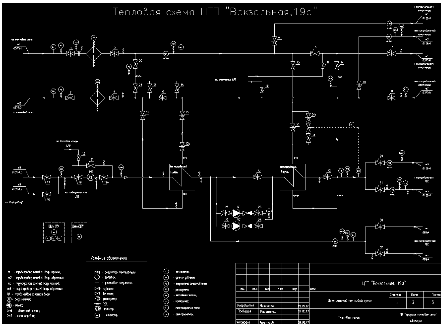
Рисунок 1.8.34 Принципиальная схема теплового пункта «Вокзальная, д. 19а»
