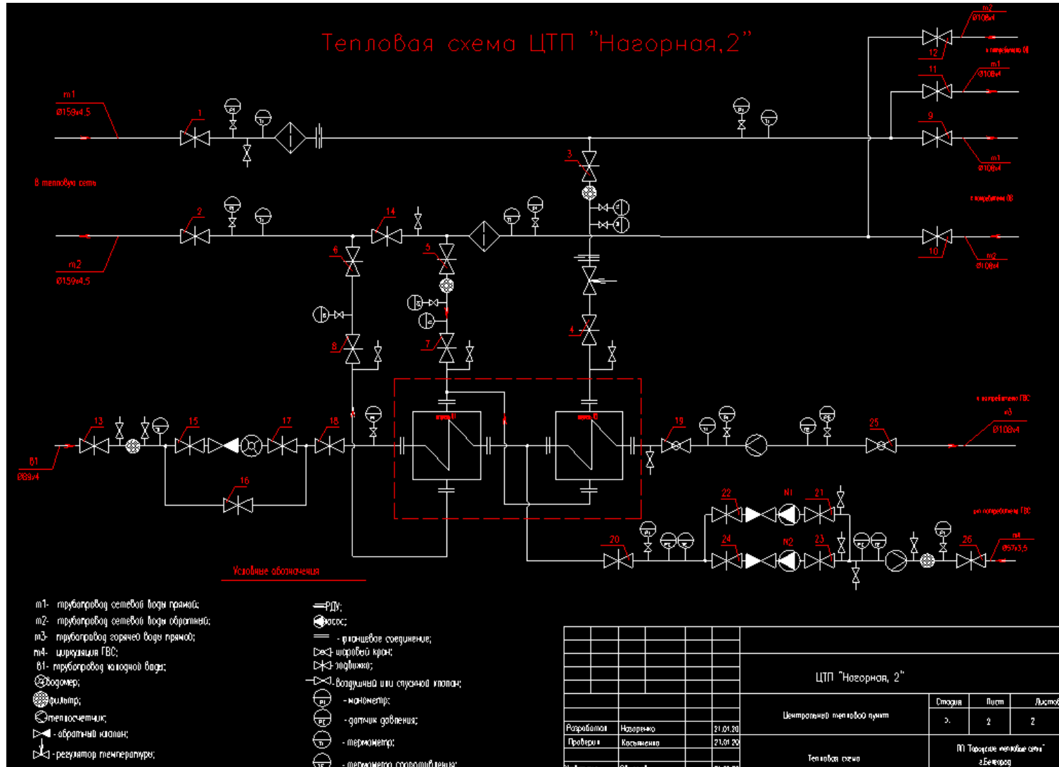
Рисунок 1.8.44 Принципиальная схема теплового пункта «Нагорная, д. 2»
