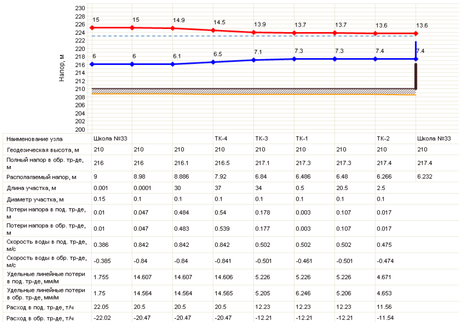
Рисунок 1.9.63 Пьезометрический график котельной «Школа, № 33»
