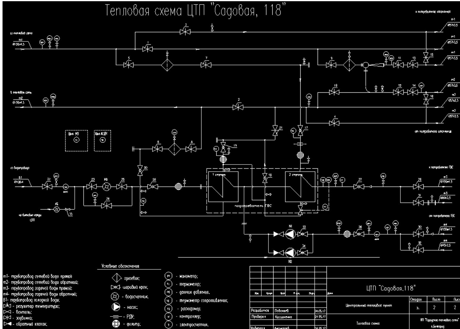
Рисунок 1.8.16 Принципиальная схема теплового пункта «Садовая, 118»
