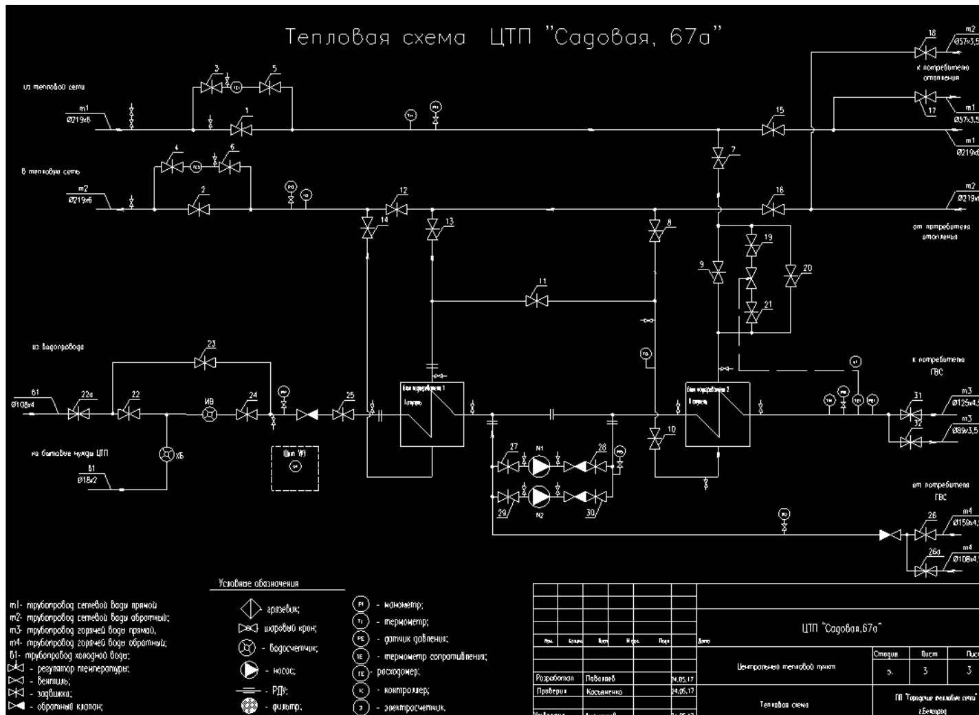
Рисунок 1.8.14 Принципиальная схема теплового пункта «Садовая, 67а»
