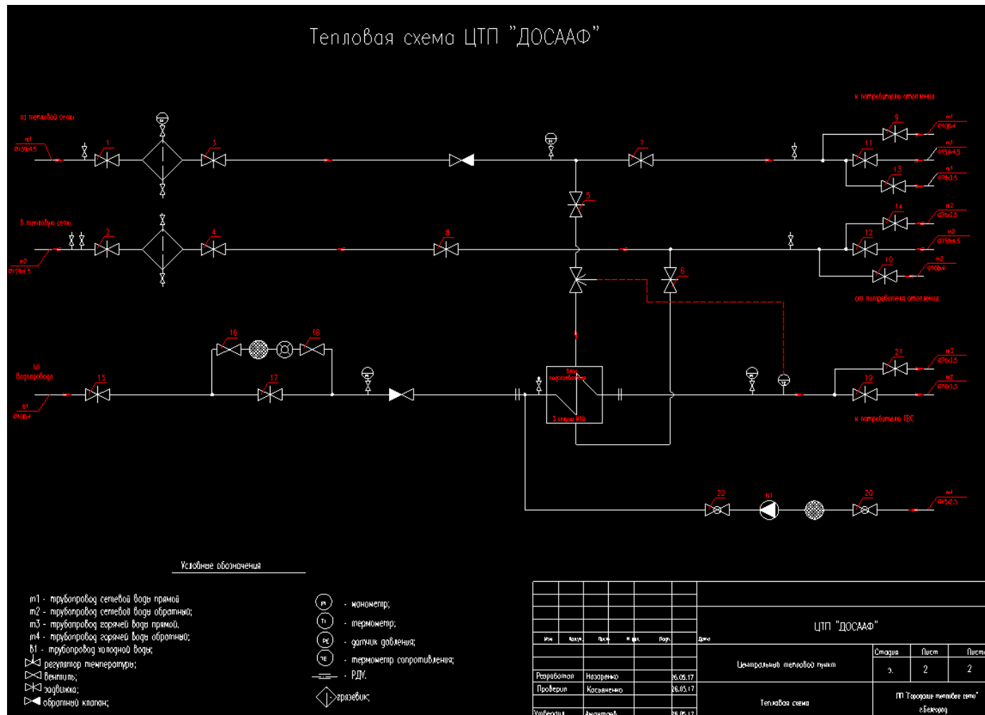
Рисунок 1.8.23 Принципиальная схема теплового пункта «ДОСААФ»
