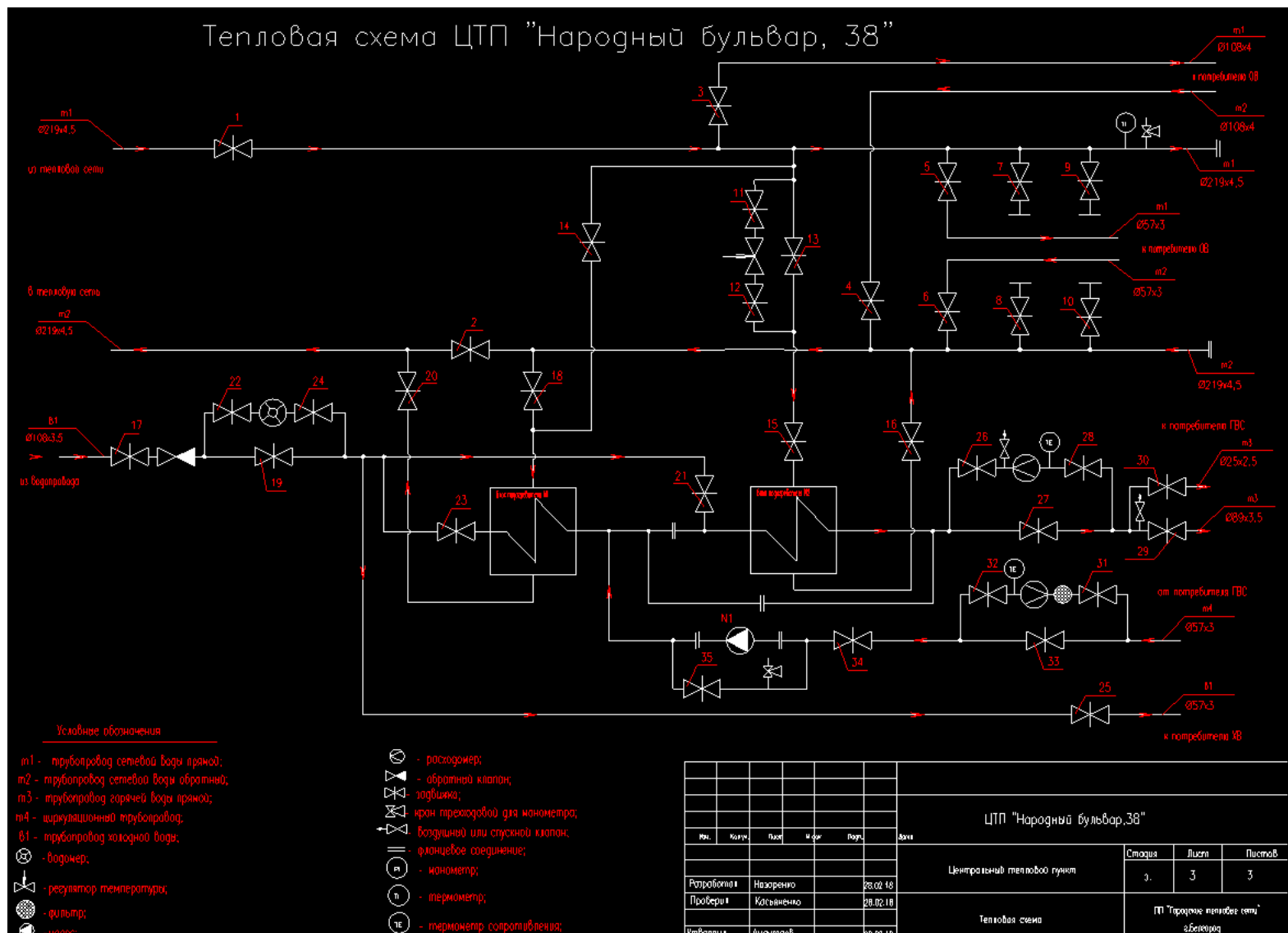
Рисунок 1.8.48 Принципиальная схема теплового пункта «Н. Бульвар, д. 38»
