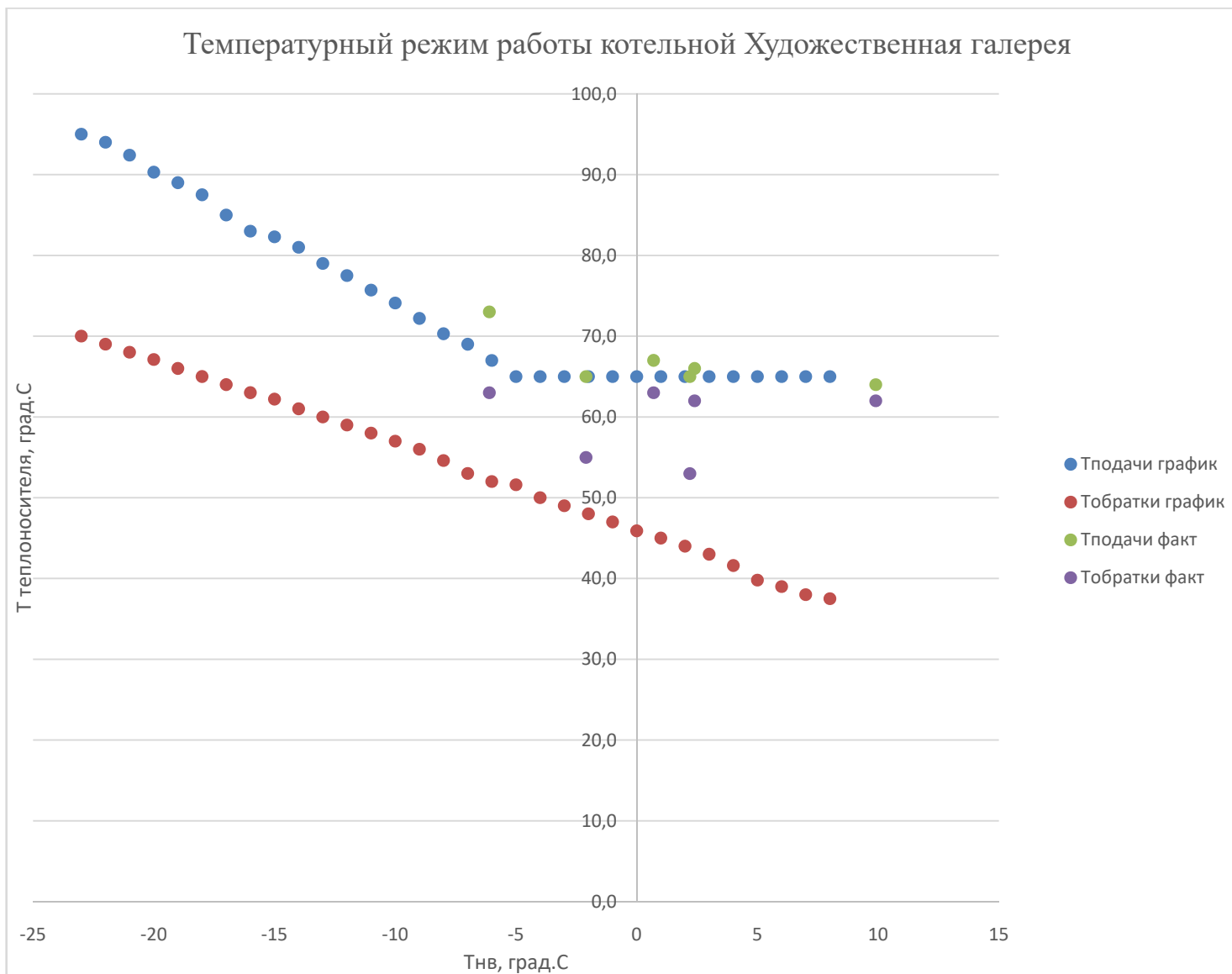
Рисунок 1.9.78 Температурный режим котельной:Художественная галерея
