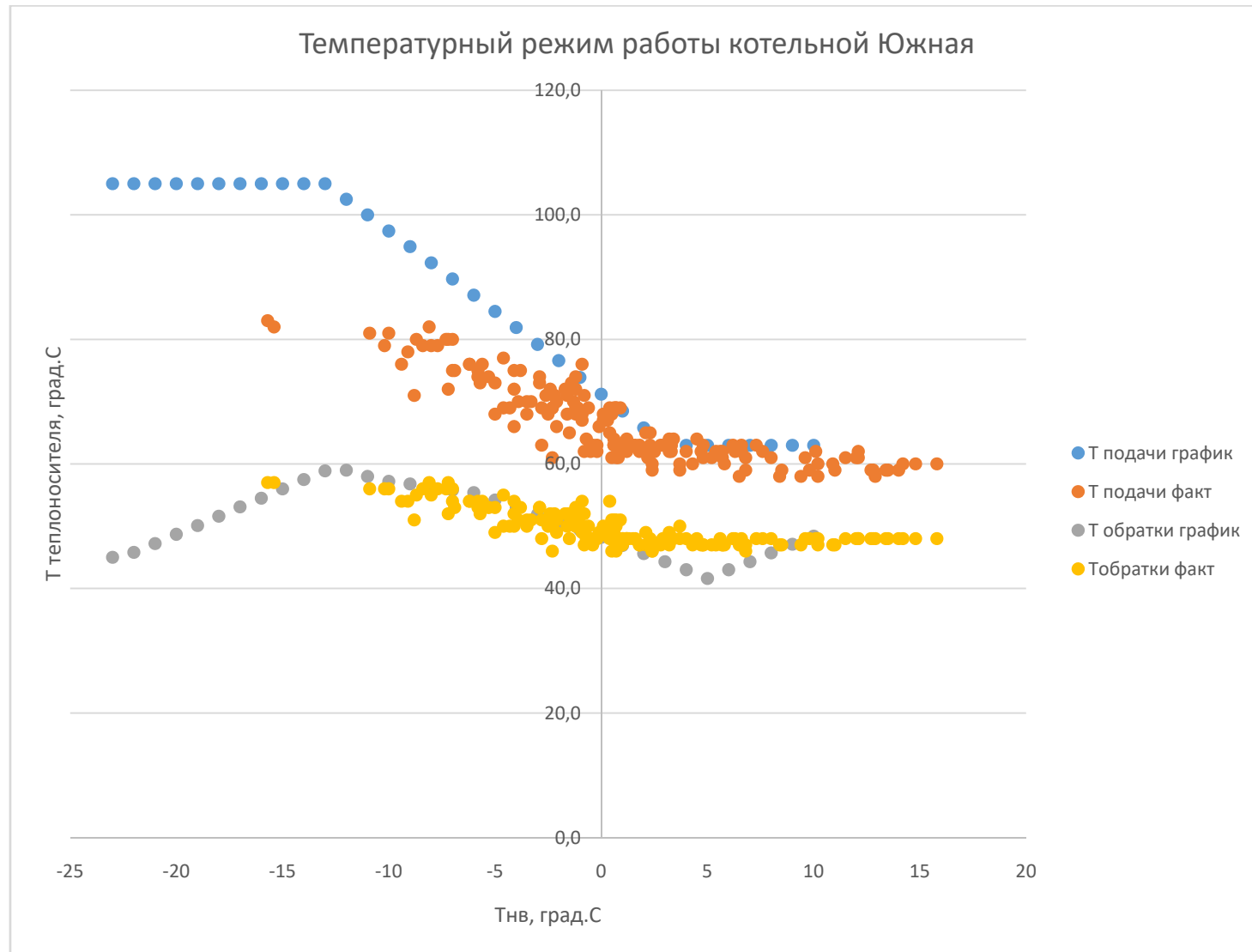
Рисунок 1.9.73 Температурные режимы котельной «Южная»
