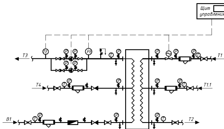
Рис. 9.2. Типовая схема подключения водоподогревателей к системе теплоснабжения
