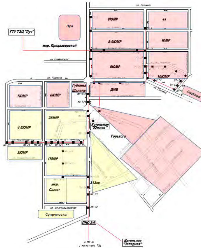
Принципиальная схема
