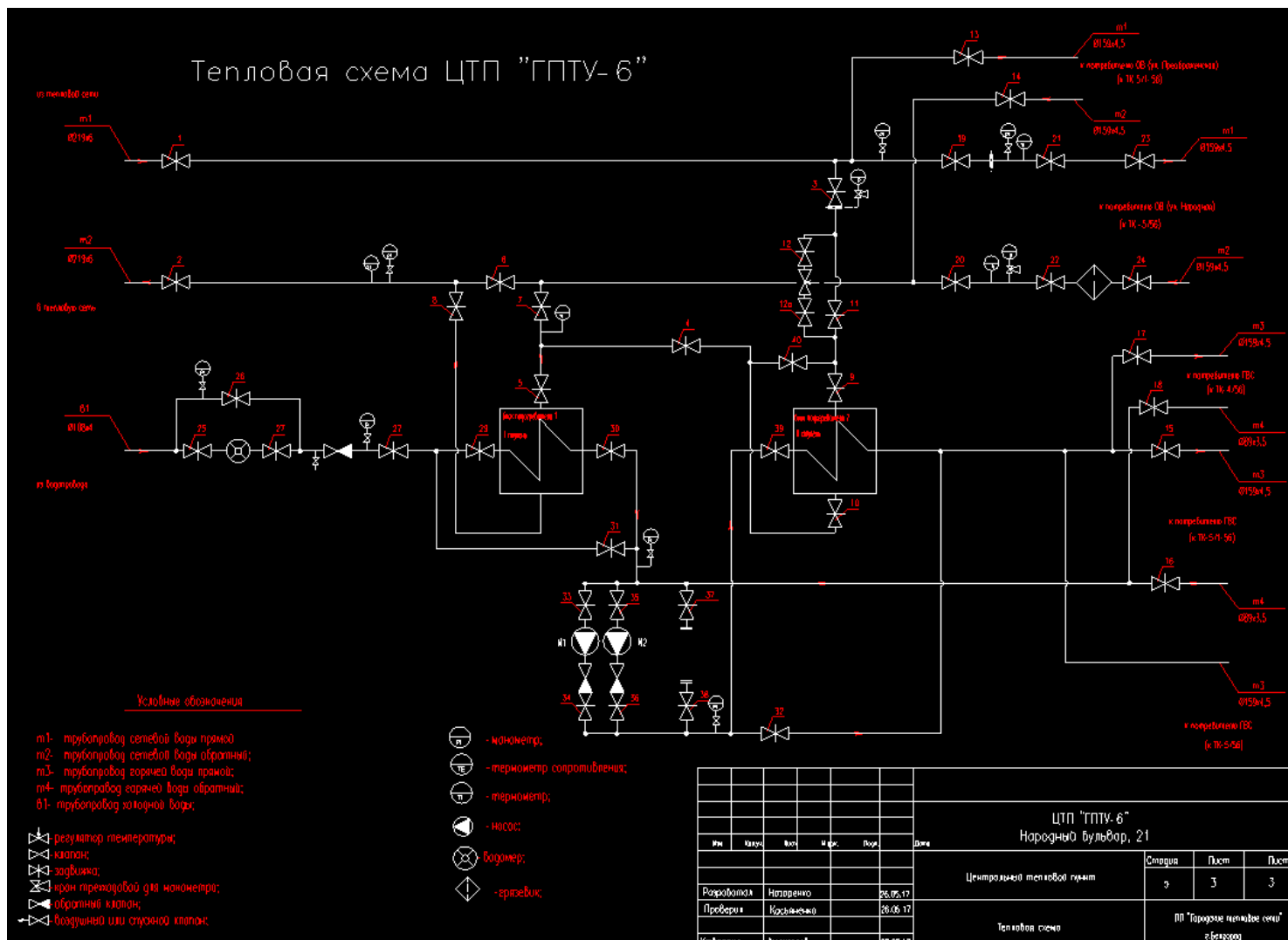
Рисунок 1.8.22 Принципиальная схема теплового пункта «ГПТУ - 6»
