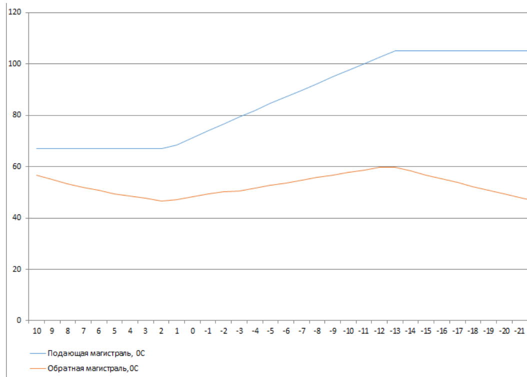
Рисунок 5.1 Температурный график «Белгородская ТЭС»
