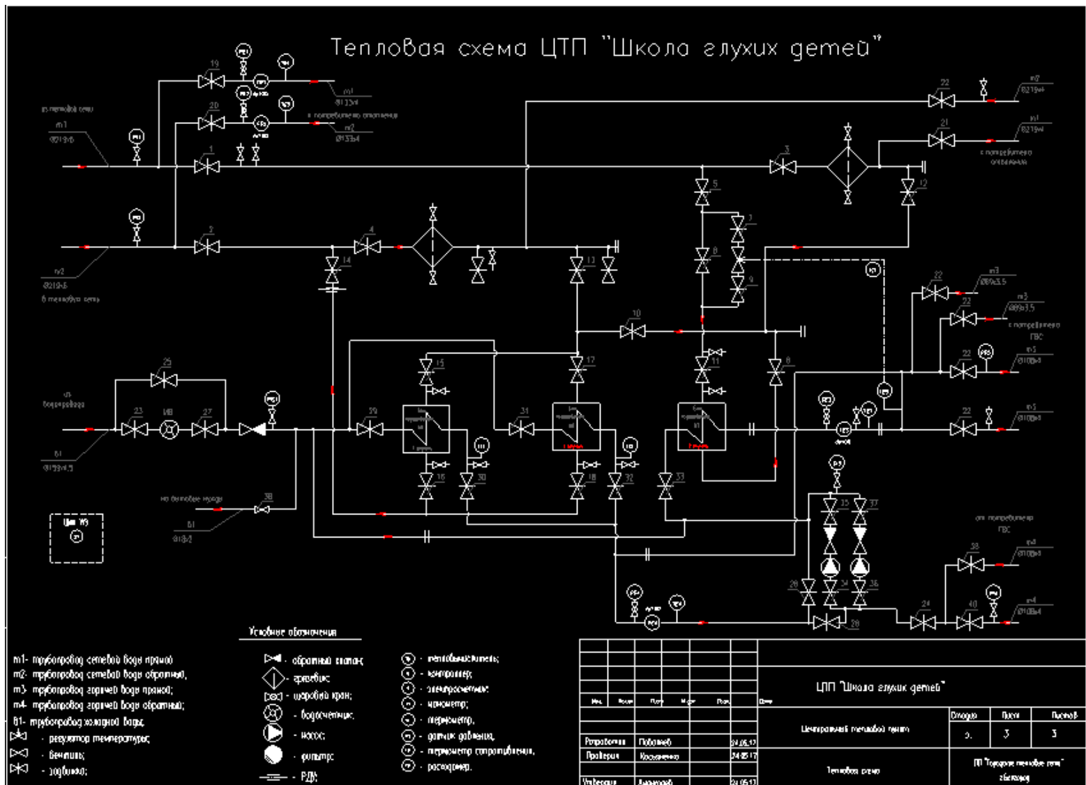
Рисунок 1.8.21 Принципиальная схема теплового пункта «Школа глухих детей»
