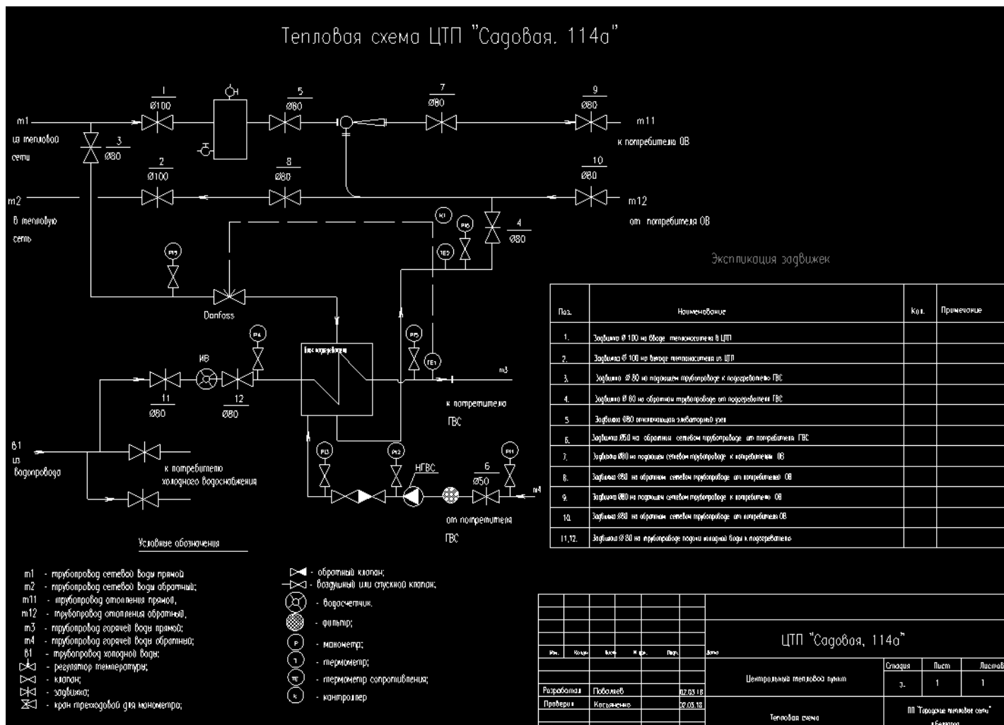
Рисунок 1.8.15 Принципиальная схема теплового пункта «Садовая, 114 а»
