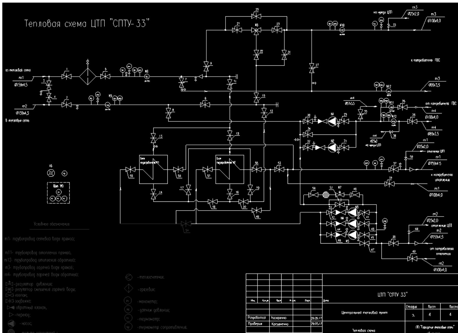
Рисунок 1.8.64 Принципиальная схема теплового пункта «СПТУ-33»
