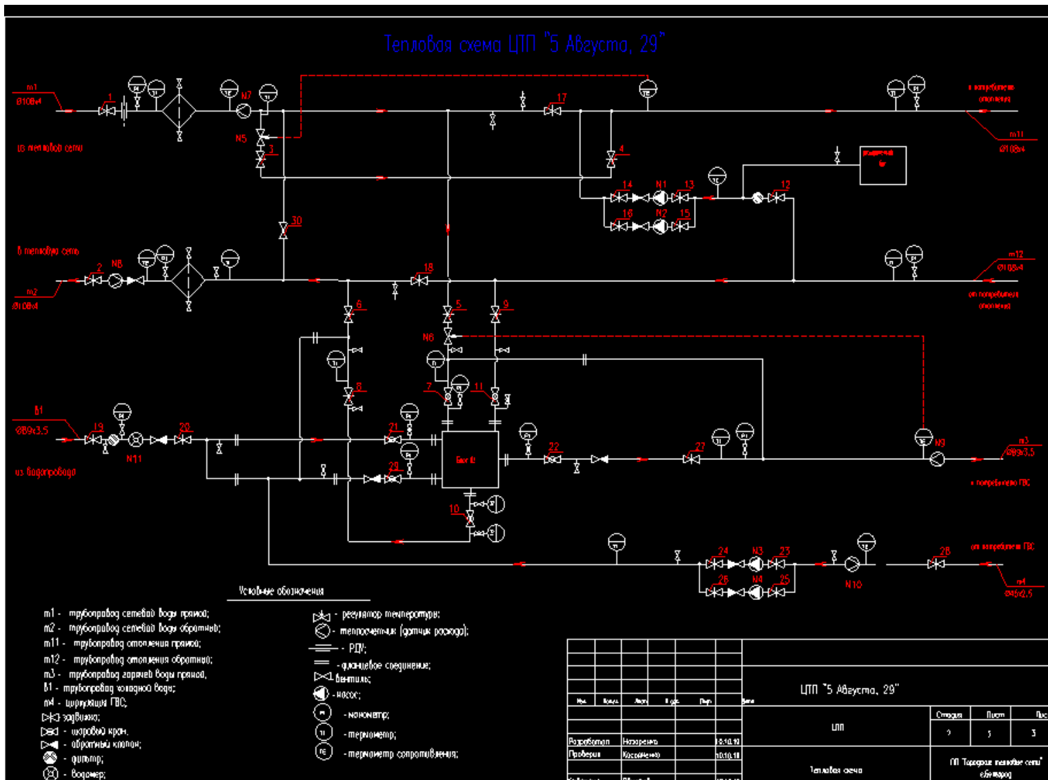
Рисунок 1.8.25 Принципиальная схема теплового пункта «5 Августа, 29»
