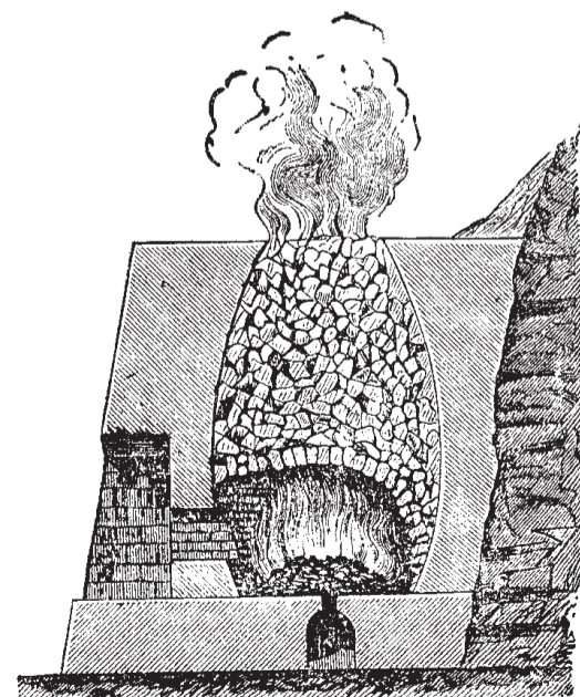
Устройство известковой печи (из словаря Брокгауза и Ефрона)
